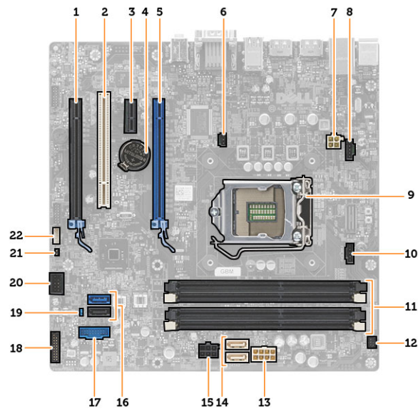
Ilustración 1. Componentes de la placa base
